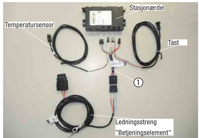
Bilde 14 ① Monter pluggforbindelser for EasyStart Web
